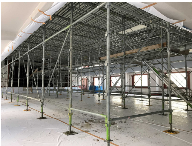
内部足場組立完了（1階）
